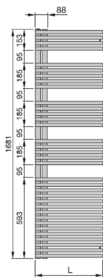
Widok z przodu, LFAR-170
