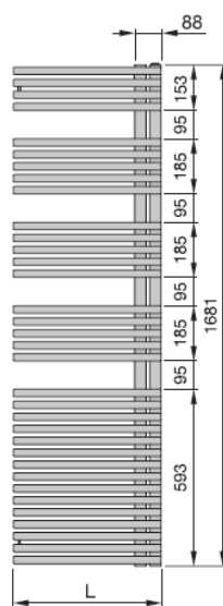
Widok z przodu, LFAL-170
