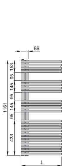
Widok z przodu, LFAR-120
