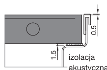
Z ramką i aluminiową kratką związaną
