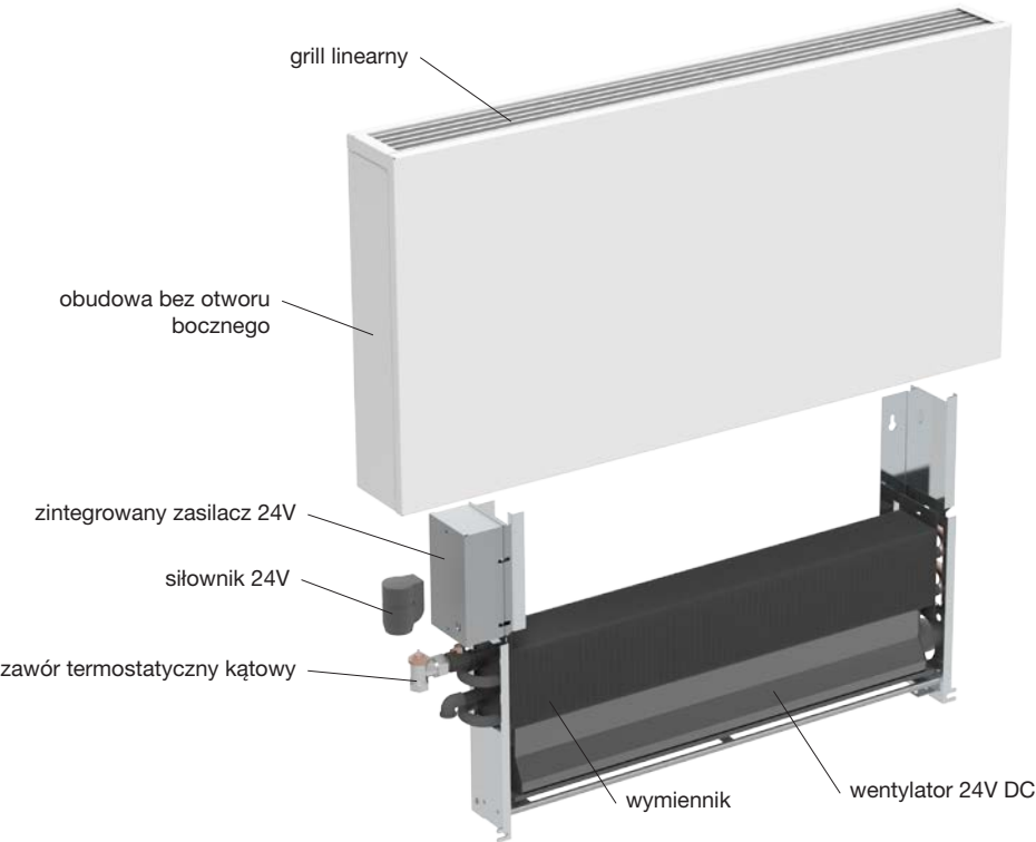
Budowa grzejnika Lateo Neo
