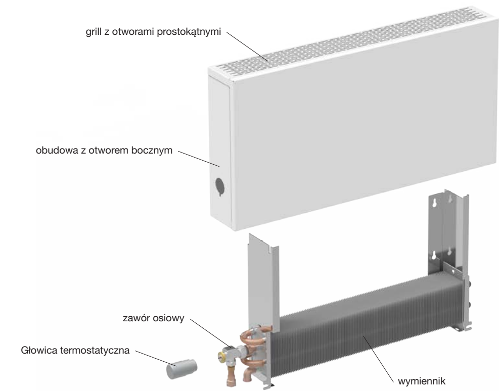
Budowa grzejnika Lateo
