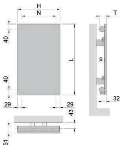
Zasilanie wodne - model ZVZA (pionowy jednowarstwowy)
