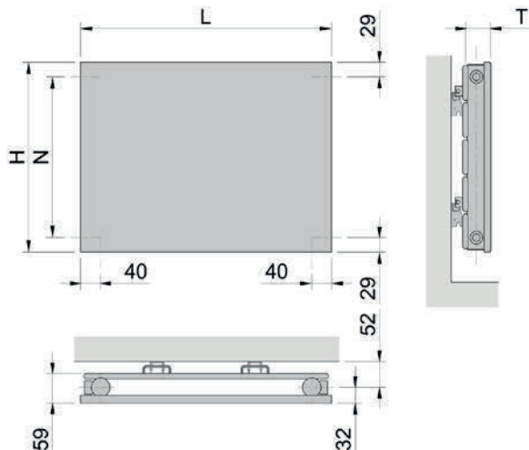
Zasilanie wodne - model ZHZAD (poziomy dwuwarstwowy)
