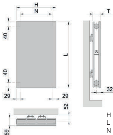
Zasilanie wodne - model ZVZAD (pionowy dwuwarstwowy)
