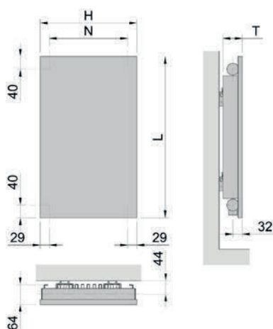
Zasilanie wodne - model ZVZLA (pionowy jednowarstwowy z lamelami)
