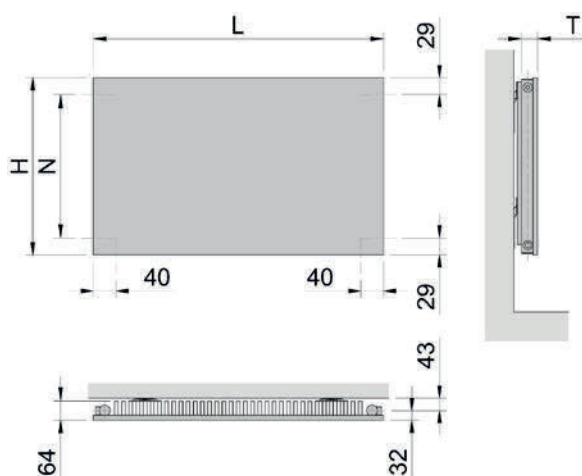
Zasilanie wodne - model ZHZLA (poziomy jednowarstwowy z lamelami)
