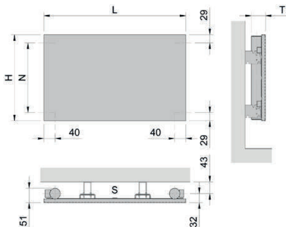
Zasilanie wodne - model ZHZA (poziomy jednowarstwowy)
